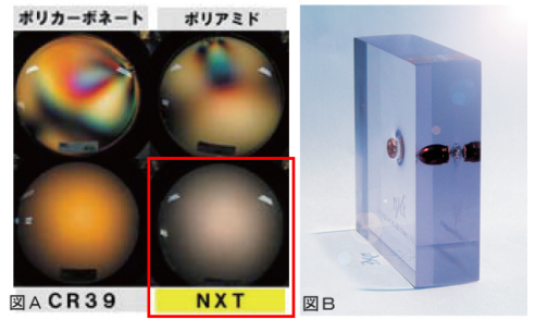
図A: 圧力をかけた後の歪み比較。NXT は歪みが残らない。 図B: マグナムの銃弾も貫通しない強度。(1m の至近距離から厚さ3cm の NXT ブロックに発砲)
